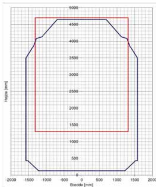
Godset læsseprofil ift. Banedanmarks læsseprofil
