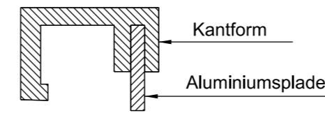
Kantprofil mål 1:1
