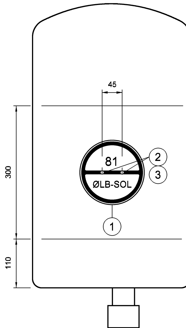
Skilt på kobler Tegning nr. KN42.196 A5911
